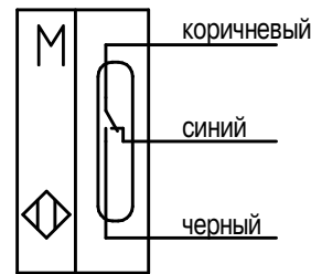
Схема подключения
